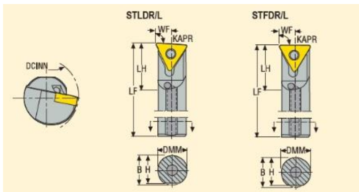
Slika 2 Za notranje struženje pri takem pritrdjevanju ploščice lahko stružimo luknje ki so le za 5 mm večje od premera držala Vir:SECO katalog
