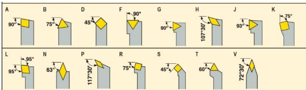
Slika 2 Tretja črka pove orientacijo rezne ploščice na držalo
