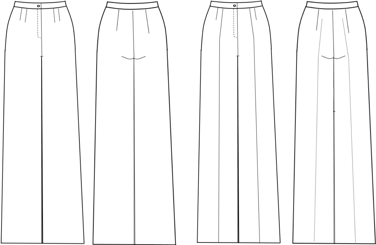
Risba št. 25: ŠIROKE HLAČE Z GUBAMI
